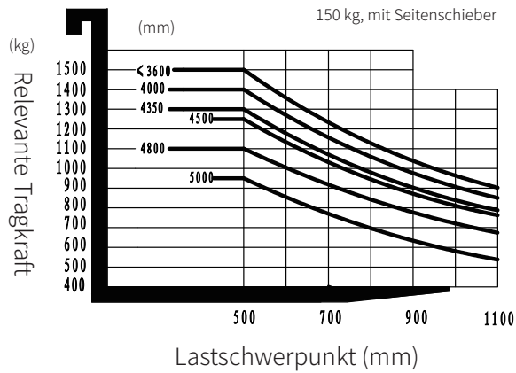
Relevante Traglasten mit Lastschwerpunkt Grafik
